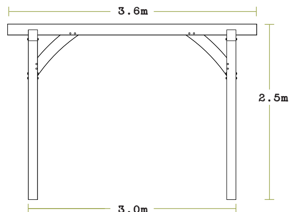
Pergola Elevation
